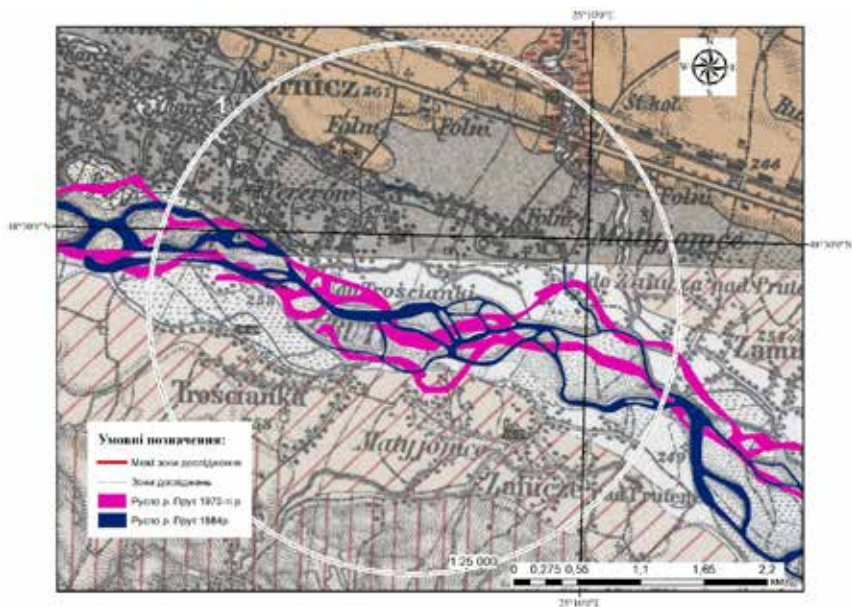
Рис. 8. Картосхема планових деформацій русла р. Прут у межах ділянки дослідження 1 на карті 1884 року
