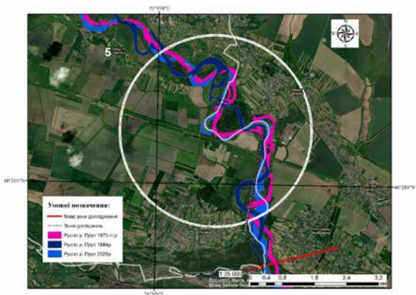
Рис. 17. Картохсхема планових деформацій русла р. Прут у межах сіл Завалля і Оршівці на знімку Sentinel L2A (ділянка 5)
